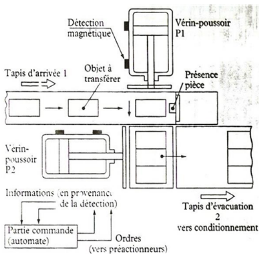
Exemple de fonctionnement d'un système séquentiel
