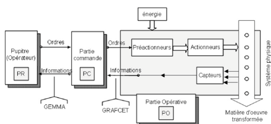
Structure d'un système automatisé
