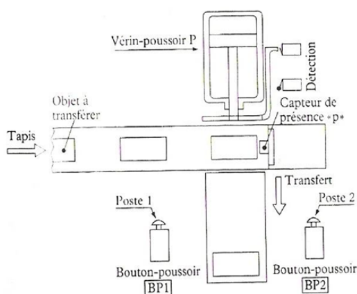
Exemple fonctionnement système combinatoire
