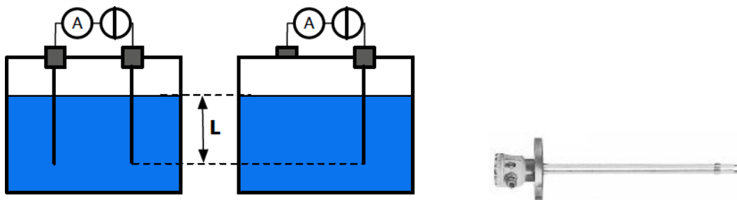
Figure V.11 : Capteurs conductimétriques
