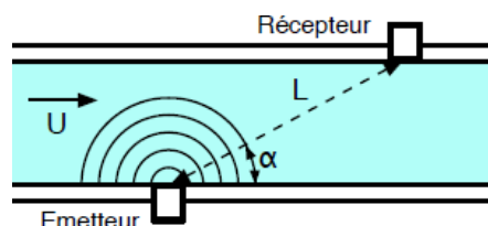
Figure V.22: Débitmètre ultrasonique
