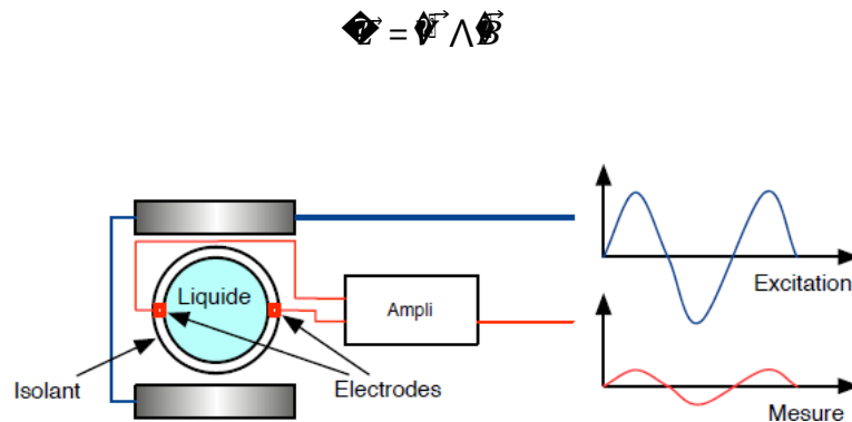
Figure V.23: Capteur électromagnétique
