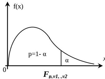
رسم 18 تعيين قيمة F يتم في الجدول يتم من خلال \nu_1 و \nu_2 و p
