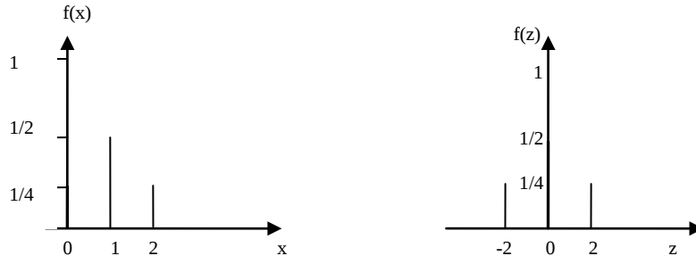
رسم 3 التمثيل البياني لدالة الكثافة للمتغيرة العشوائية المنقطعة
