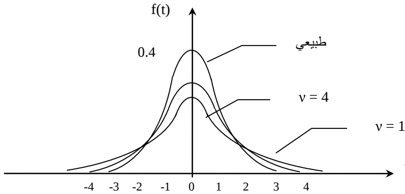
رسم 16 تدرج منحني ستيودنت حسب درجة الحرية
